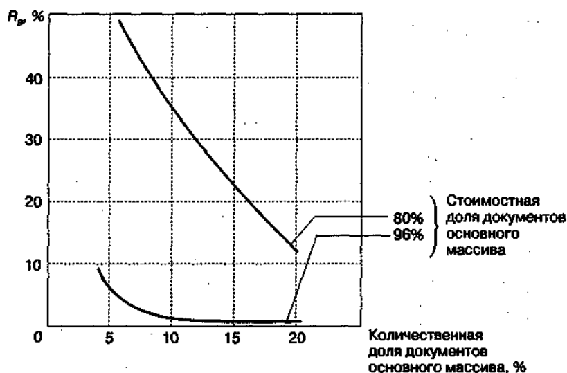
Рис. 3.1. Риск выборки R_p для метода основного массива при уровне существенности s = 2\%
